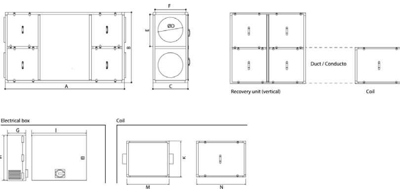
Διαστάσεις σειράς DOMEX EEC (κατακόρυφη τοποθέτηση)
