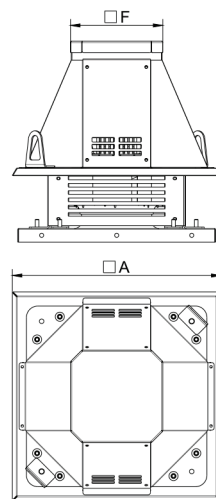
Διαστάσεις CTH3-A (mm)
