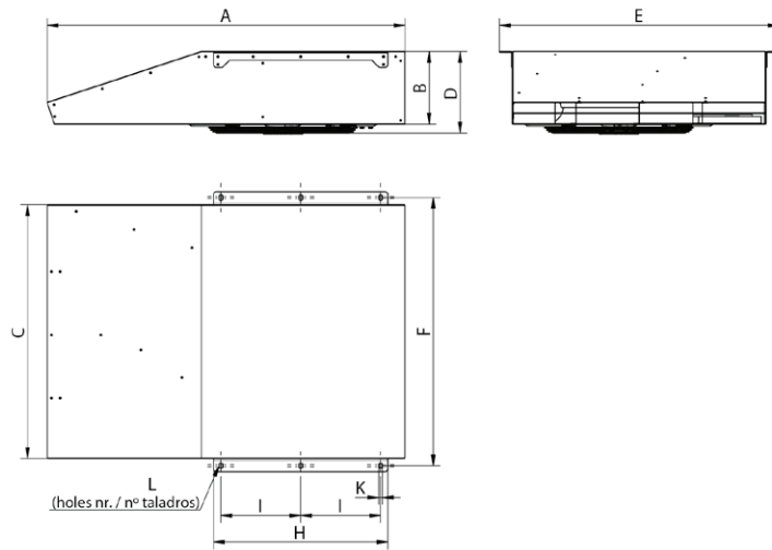
Διαστάσεις SYBILO
