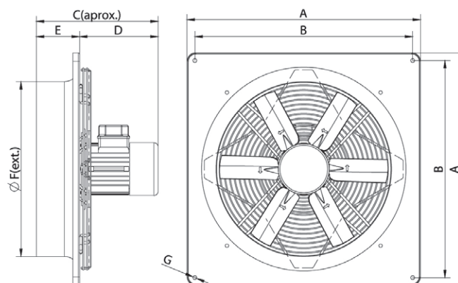
Διαστάσεις ΗJBMX (mm)
