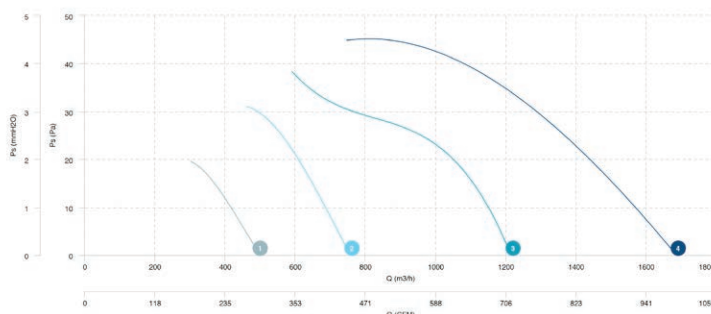
1 ΗJEM 20 M4 2 ΗJEM 25 M4 3 ΗJEM 30 M4 4 ΗJEM 35 M4
