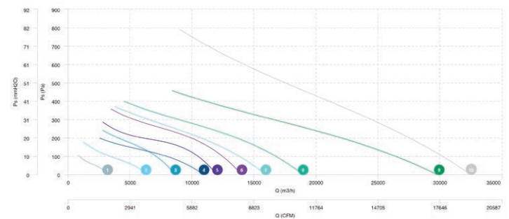
2 HH 45 T4 0,37kW 3 HH 56 T4 0,55kW 4 HH 56 T4 0,75kW 5 HH 56 T4 1,1kW 6 HH 63 T4 1,1kW 7 HH 71 T4 1,1kW 8 HH 71 T4 1,5kW 9 HH 90 T4 3kW 10 HH 90 T4 5,5kW
