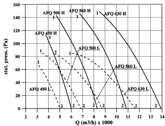
AFQ 4 πόλοι 400 V / 50Hz 450 - 630
