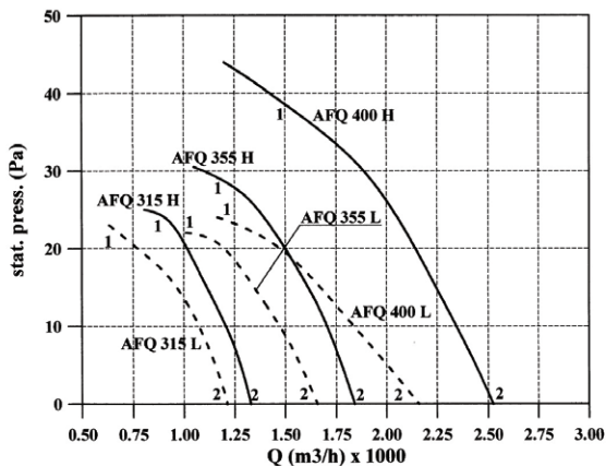
AFQ 6 πόλοι 400 V / 50Hz 315 - 400
