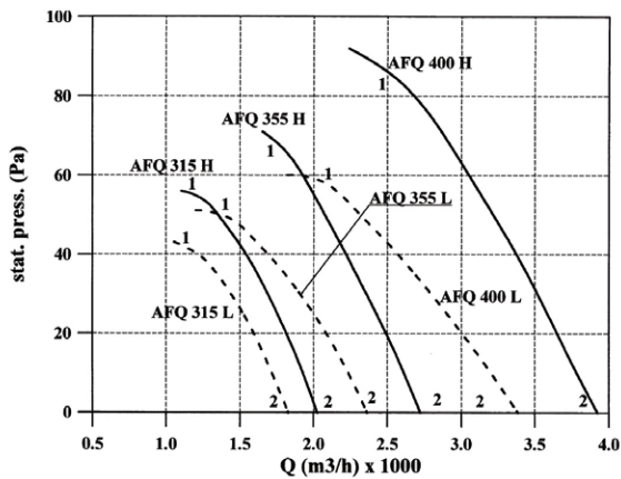
AFQ 4 πόλοι 400 V / 50Hz 315 - 400
