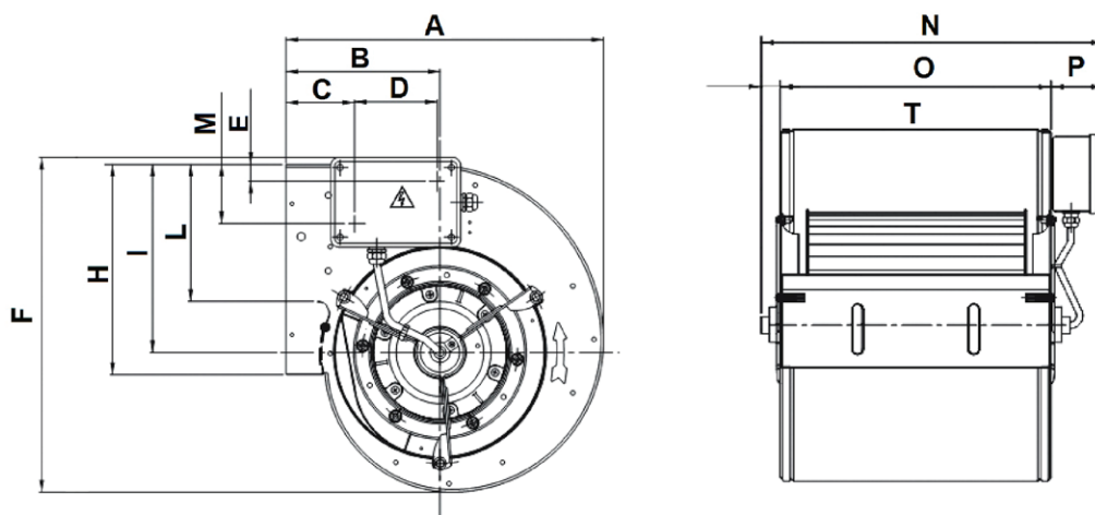
Dimensions DDM 6 3V (mm)
