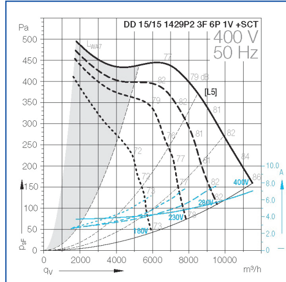
DD 15/15 2.200 6P-1V/400V
